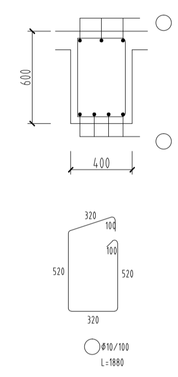
A-A KESİTİ
